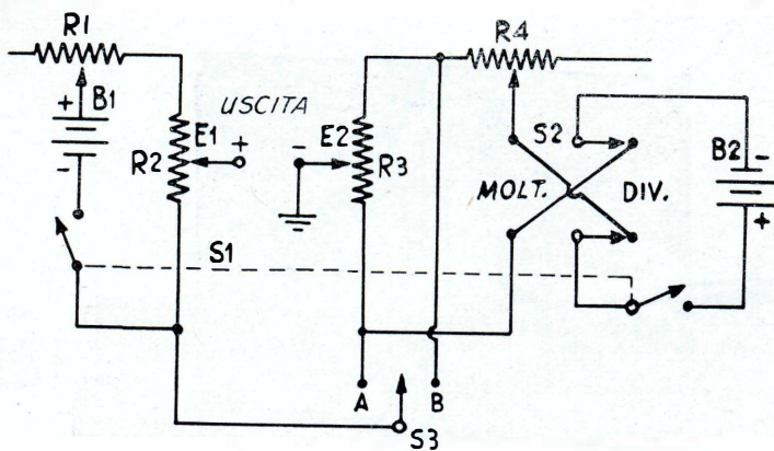
Schema elettrico del modello funzionale di regolo calcolatore elettron.
