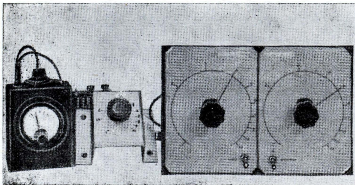
Uso dell'indicatore di azzeramento in luogo del voltmetro a valvola (schema in figura 3, vedere testo).
