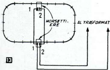
Collegamento di un altro elemento di rotaia munito di morsettiere per fornire correnti anche ai punti più distanti dalle rotaie.
