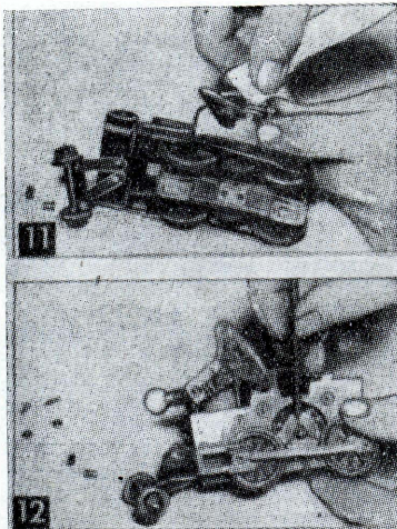
Fig. 11. - Gli alloggiamenti delle spazzole debbono essere mantenuti ben puliti per permettere alle spazzole di muoversi liberamente in essi, in caso contrario potrebbe risultare un cattivo contatto tra le spazzole ed il collettore, da cui deriverebbe un eccessivo scintillamento ed un surriscaldamento che potrebbe danneggiare il rotore. Per pulire gli alloggiamenti delle spazzole, farvi scorrere dentro un leghetto di un fiammifero, su cui sia stato avvolto un batuffoletto di cotone.
