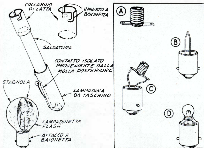
Figura di sinistra - Come la lampada da taschino deve essere modificata per funzionare come portafash, con attacco a baionetta.
