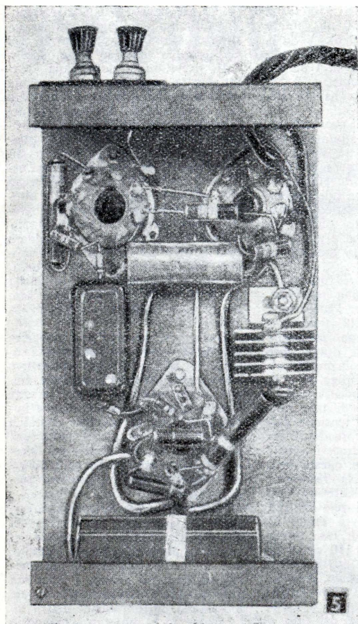
Il ricevitore a fotocellula, visto dal di sotto; notare i pochi e semplici collegamenti necessari.
