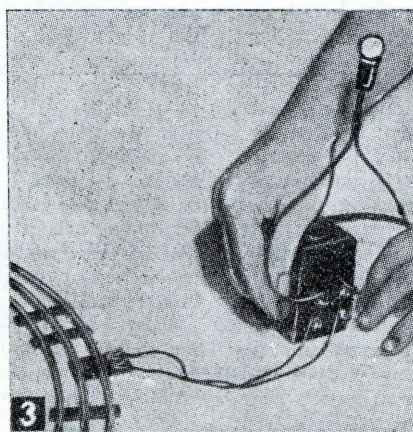
Fig. 2. - Prova per constatare la presenza della corrente a bassa tensione alla morsetteria fissata ad uno degli elementi di rotaia. La lampada cercaguasti utile per queste prove può essere realizzata utilizzando alcuni dei materiali impiegati per i festoni luminosi degli alberi di Natale. Fig. 3. - Controllo al secondario del trasformatore, per vedere se in questo punto sia presente la tensione che poi, attraverso un conduttore viene inviata alla morsetteria e di là si propaga in tutte le rotaie. I terminali inferiori che si possono notare sul trasformatore sono quelli che forniscono la tensione a tutti gli accessori dell'impianto ferroviario. Se il trasformatore appare in buone condizioni collegare ad esso il conduttore che porta corrente alla morsetteria; se la lampada cercaguasti si spegne, è segno che un cortocircuito è presente in qualche parte. Fig. 4. Controllo dell'elemento di rotaia al quale è fissata la morsetteria, per vedere se vi siano dei cortocircuiti. La prova in tal senso va condotta con la lampada cercaguasti collegata direttamente ai terminali del trasformatore.
