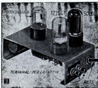
Complesso ricevitore a fotocellula, montato su di uno chassis auto-costruito.
