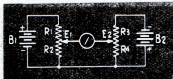
Circuito di base per il regolo calcolatore elettronico; vedere testo per la completa spiegazione dei principi applicati.
