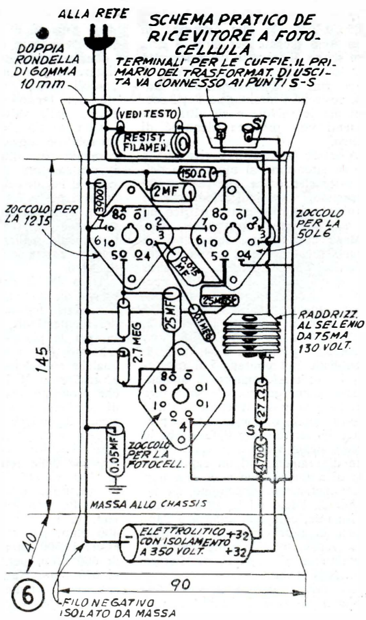
Il ricevitore a fotocellula, visto dal di sotto; notare i pochi e semplici collegamenti necessari.
