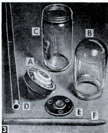
A) portalampade impermeabile. B) globo. C) barattolo di vetro che può servire come globo. D) tubo di acciaio brunito. E) flangia con filettatura centrale adatta al tubo. F) tondino appuntito di legno duro.
