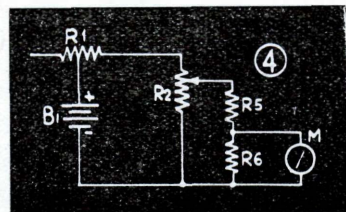
Schema basilare per il circuito per l'estrazione delle radici dai numeri.
