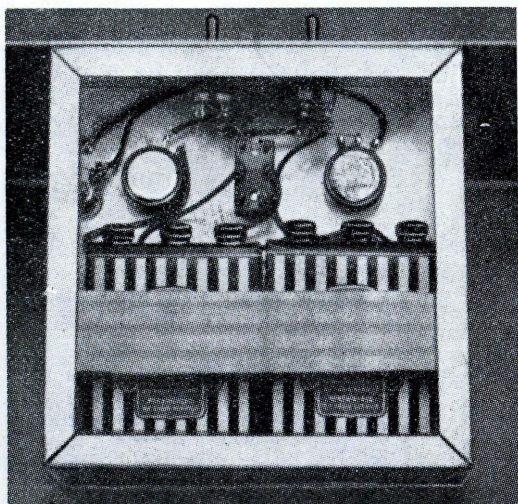
Il calcolatore visto dal di sotto dello chassis, i collegamenti sono eseguiti da punto a punto.
