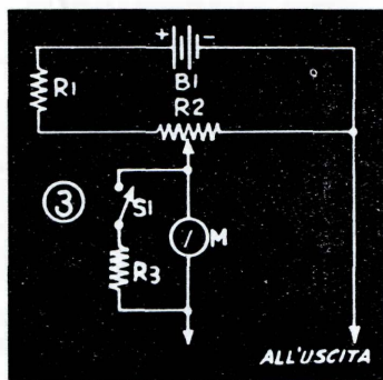
Schema di impiego di un indicatore di azzerramento in luogo di un voltmetro a valvola.
