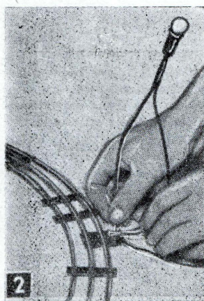
Fig. 2. - Prova per constatare la presenza della corrente a bassa tensione alla morsetteria fissata ad uno degli elementi di rotaia. La lampada cercaguasti utile per queste prove può essere realizzata utilizzando alcuni dei materiali impiegati per i festoni luminosi degli alberi di Natale. Fig. 3. - Controllo al secondario del trasformatore, per vedere se in questo punto sia presente la tensione che poi, attraverso un conduttore viene inviata alla morsetteria e di là si propaga in tutte le rotaie. I terminali inferiori che si possono notare sul trasformatore sono quelli che forniscono la tensione a tutti gli accessori dell'impianto ferroviario. Se il trasformatore appare in buone condizioni collegare ad esso il conduttore che porta corrente alla morsetteria; se la lampada cercaguasti si spegne, è segno che un cortocircuito è presente in qualche parte. Fig. 4. Controllo dell'elemento di rotaia al quale è fissata la morsetteria, per vedere se vi siano dei cortocircuiti. La prova in tal senso va condotta con la lampada cercaguasti collegata direttamente ai terminali del trasformatore.
