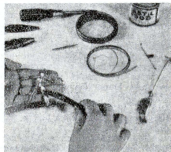
Applicazione dello stucco plastico al di sopra ed in mezzo allo scheletro in filo di ferro.
